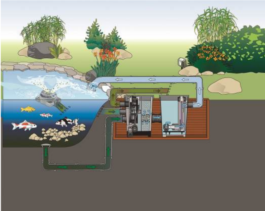
Der ProfiClear Premium Compact EGC bietet eine hohe Leistung bei kompakten Abmaßen. (Bild: OASE GmbH).
